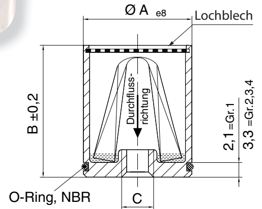
Ausführung mit O-Ring
